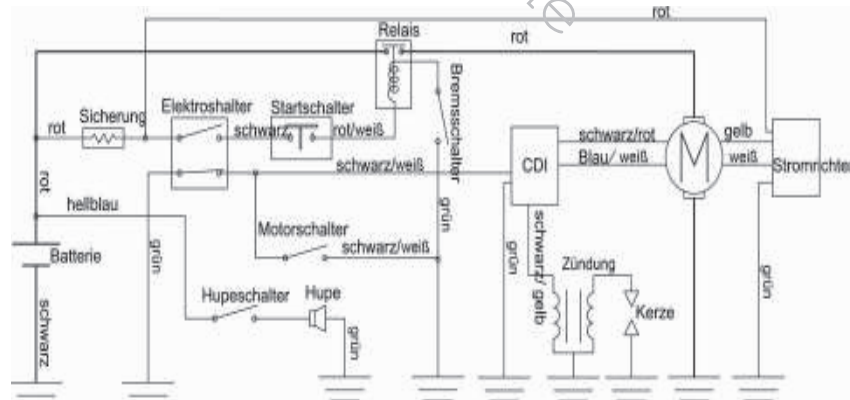
SCHALTPLAN-KXD708:
