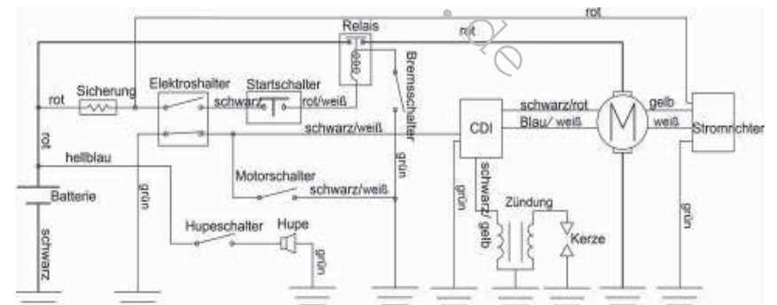
SCHALTPLAN-KXD608:
