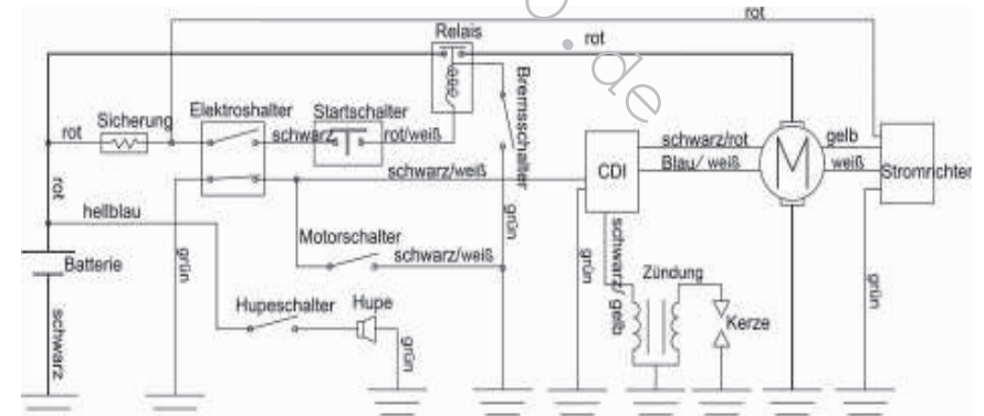
SCHALTPLAN-KXD612:
