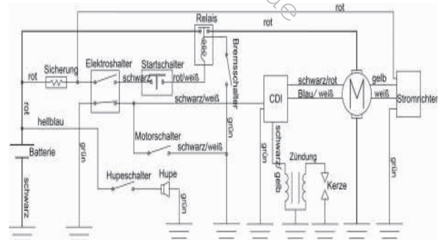
SCHALTPLAN-KXD607:
