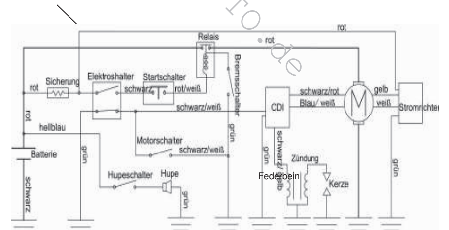
SCHALTPLAN-KXD609:
